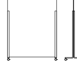
Paretina divisoria su ruote H145 Partition H145 on castors
